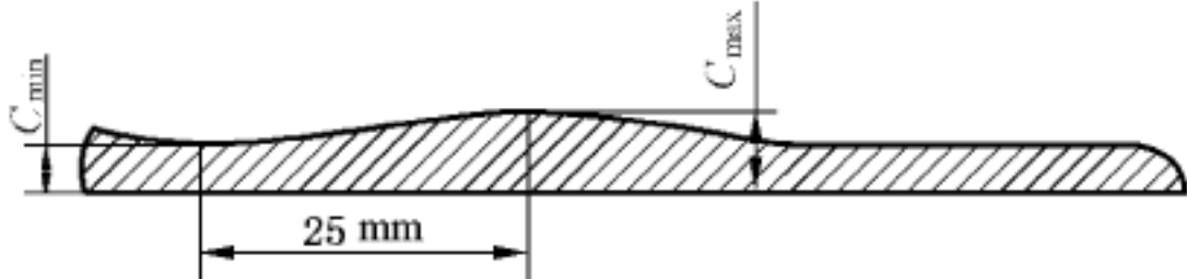
图 4 焊缝表面余高差示意图
