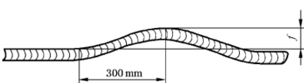
图 3 焊缝边缘直线度示意图
