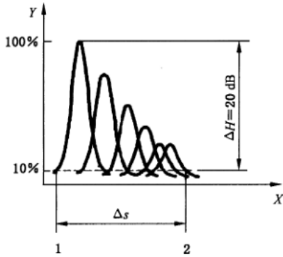
c) 回波动态波形
