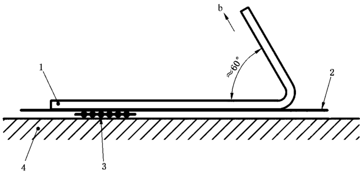
b) 从网格上撕离胶带前胶带的位置
