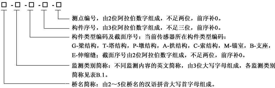
图 3 桥梁监测点编号命名规则
