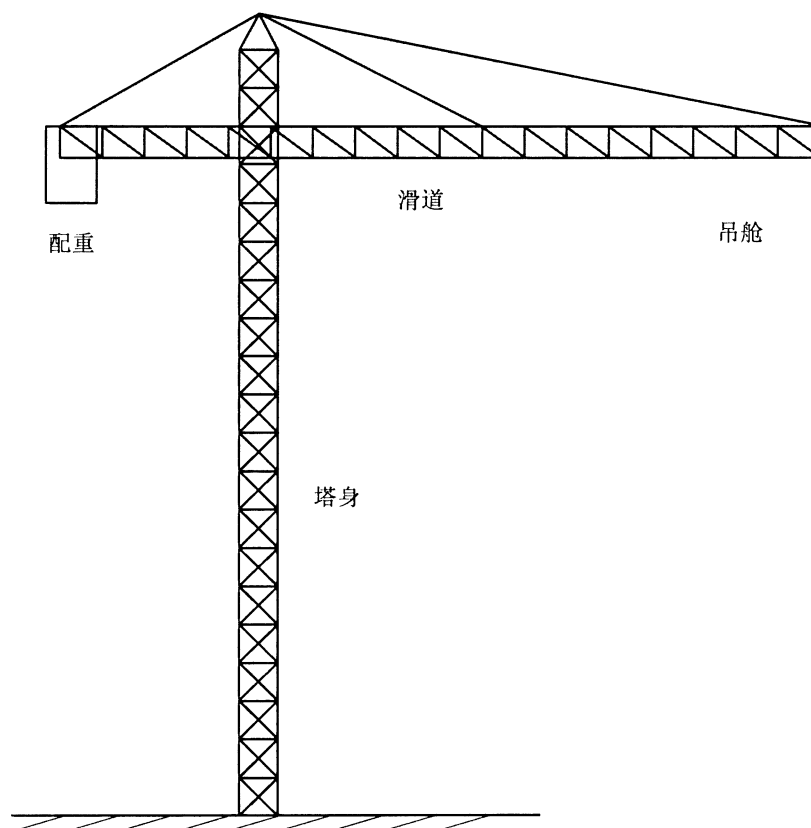
图 B.1 空中滑道示意
