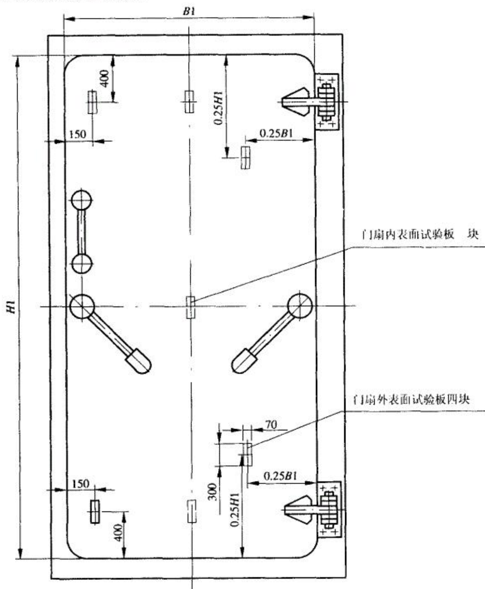
图 3.4.4-6 试验板布置图
