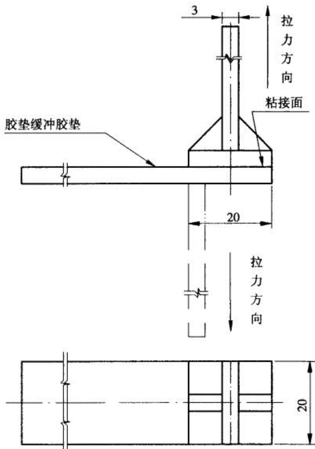
图 3.4.6-2 剥离强度检验试件图
