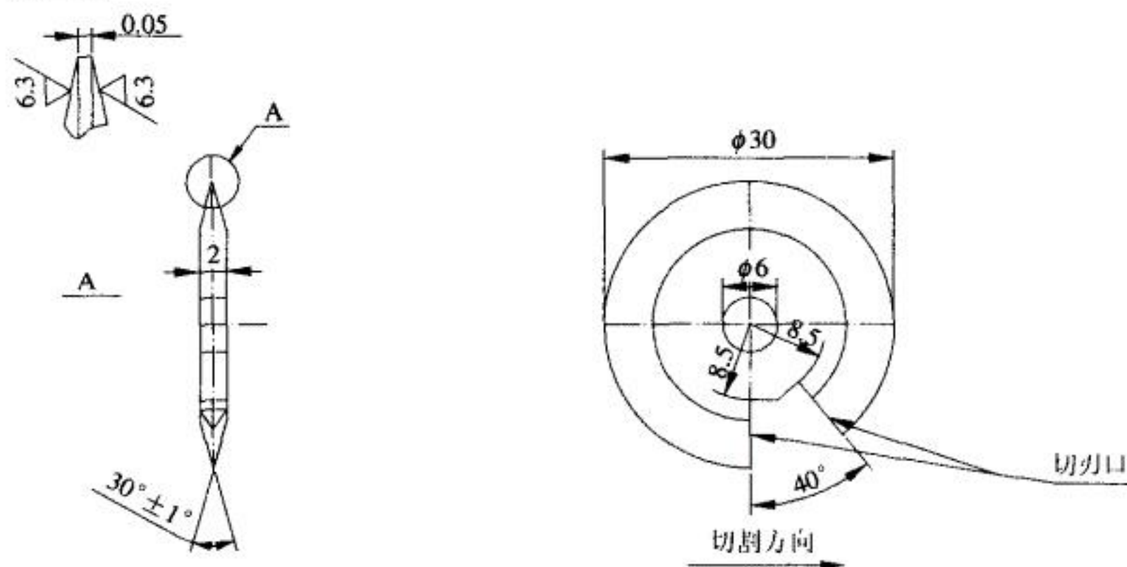
a) 单刃刀具
