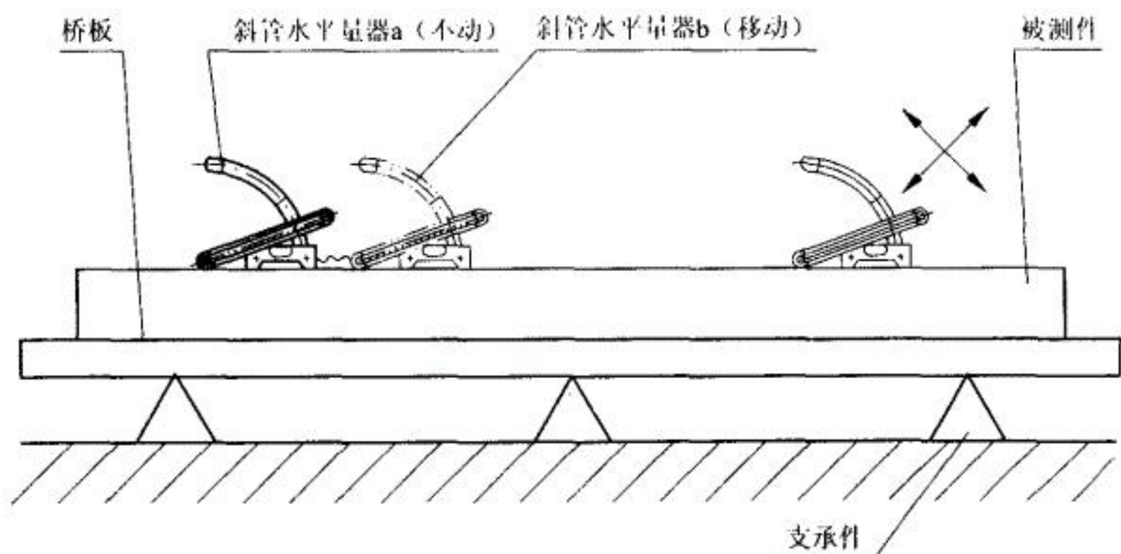
图 3.4.4-3 平面度测量方法二示意图
