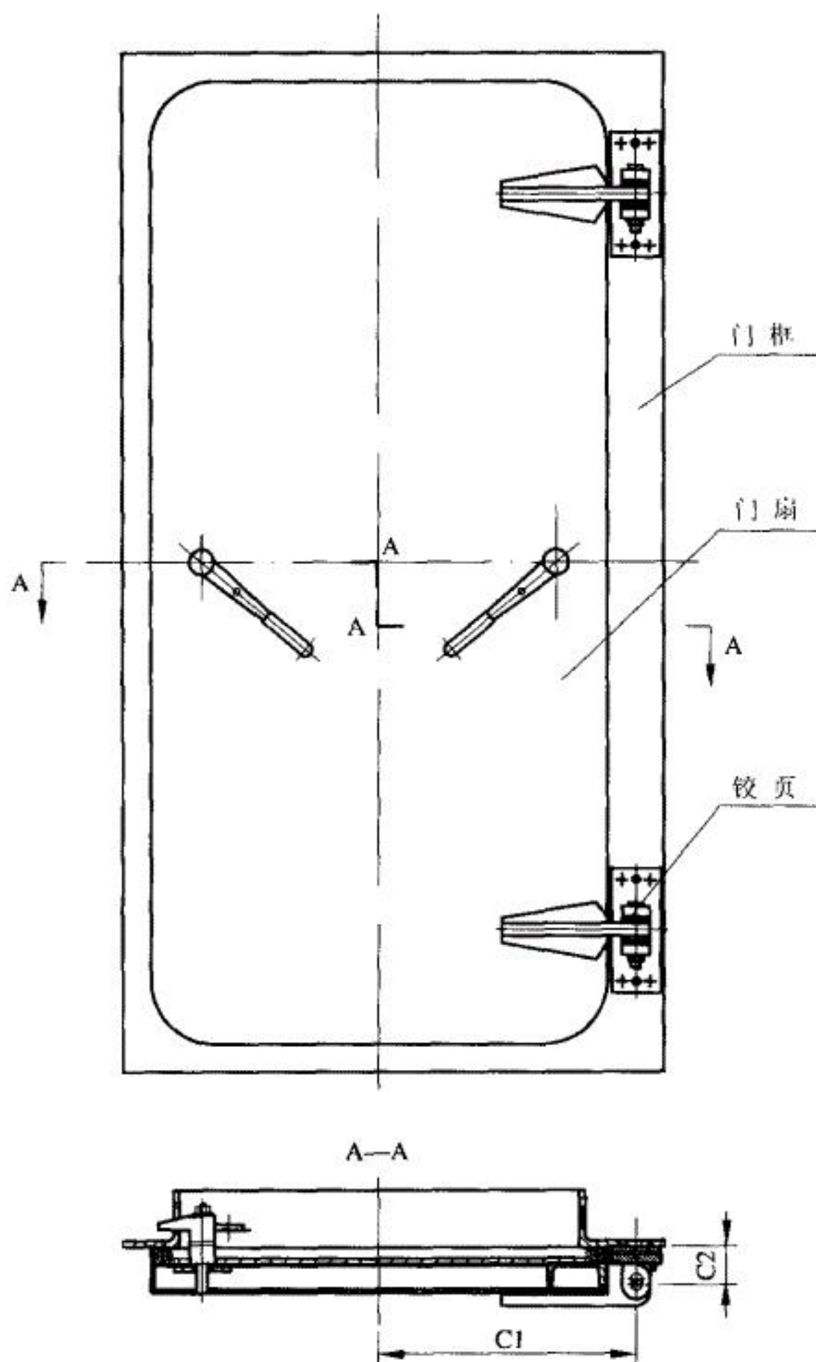
附图 3.4.4-1 铰页与门框、门扇配合图
