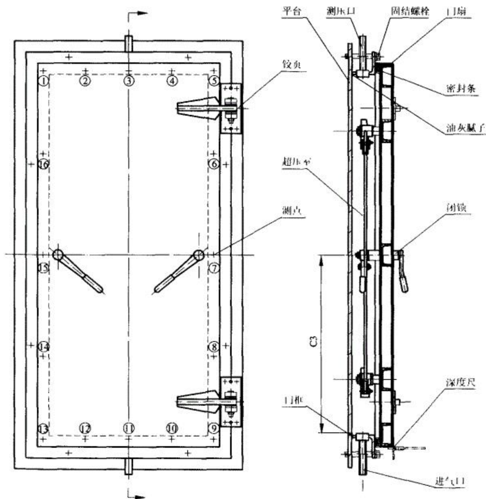
图 3.4.3-1 漏气量测量装置
