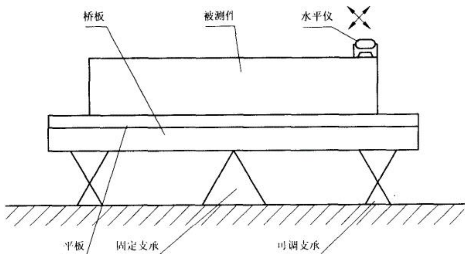
图 3.4.4-2 平面度测量方法一示意图
