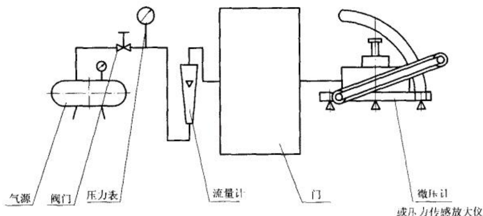
附图 3.4.3-2 测量气路图
