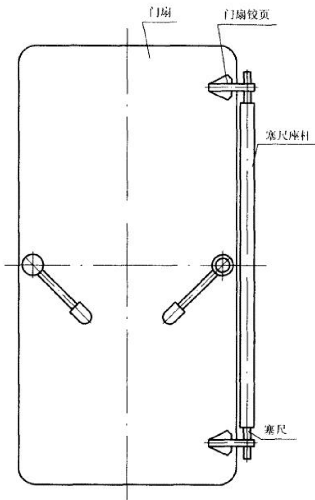
图 3.4.4-4 门扇铰页孔同轴度检测图
