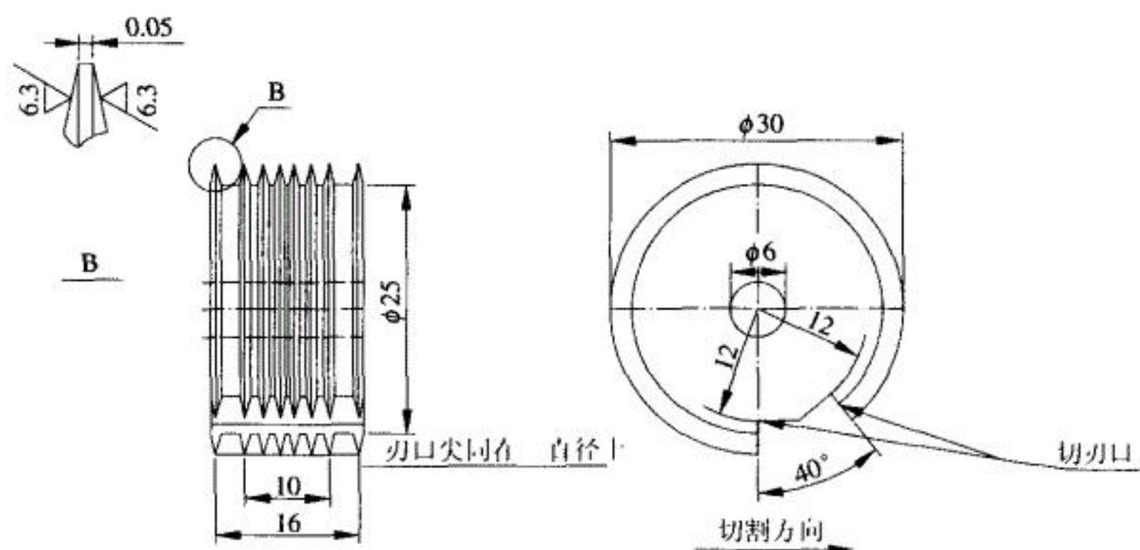
b) 多刃刀具
