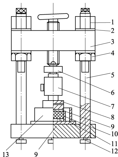
图 4.19.3-3 岩石膨胀压力试验仪
