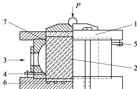
图 4.34.2 侧压力仪试验装置示意图
