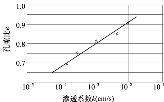
图 4.24.3-2 孔隙比 e 与渗透系数 k 关系曲线
