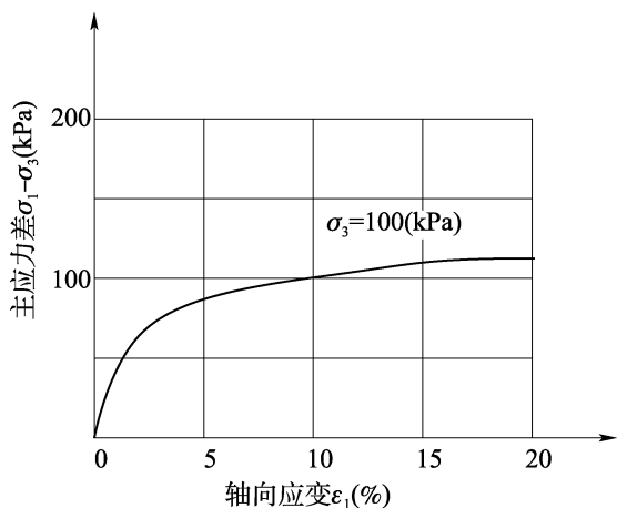
图 4.26.5-2 主应力差与轴向应变关系曲线
