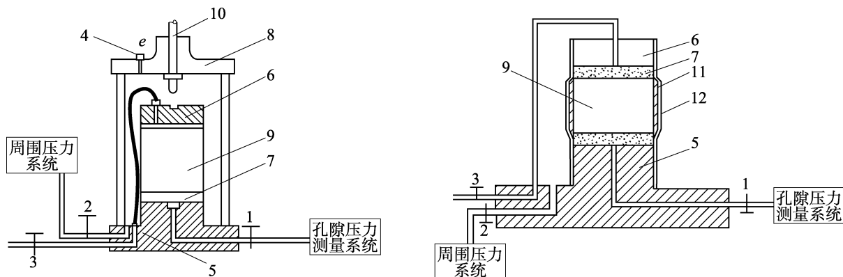
(a) 各向等压消散试验装置
