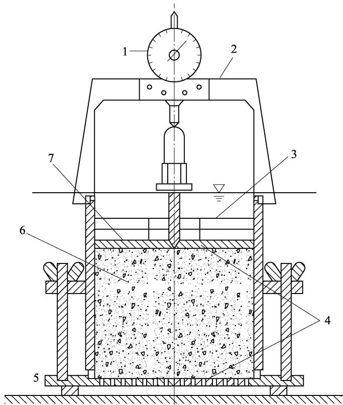
图4.22.5 浸水膨胀试验装置
