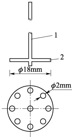
图 4.32.2-1 搅拌器示意图
