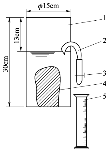
图 4.11.3 排液筒装置示意图
