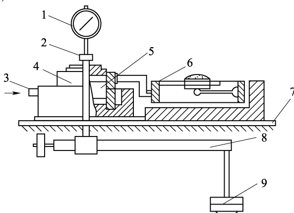
图 4.30.2 应变控制式直剪仪结构示意图
