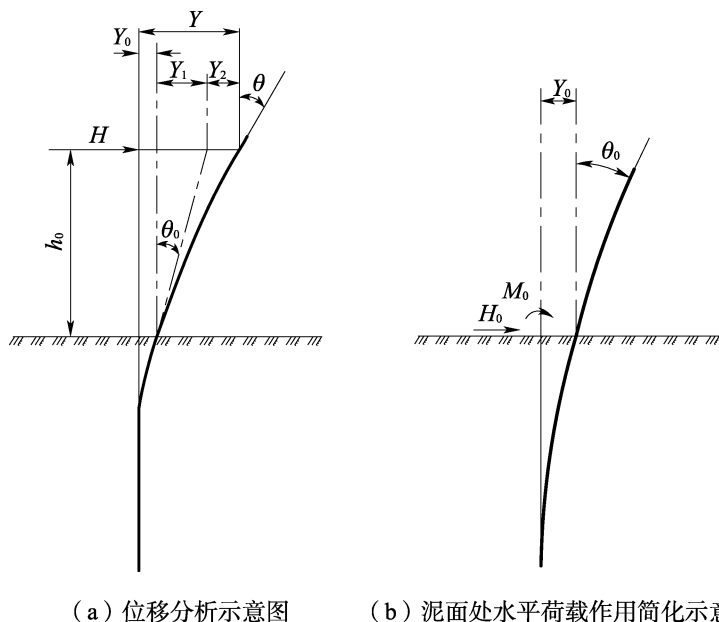
图 E.0.1 弹性长桩在水平荷载作用下的位移分析示意图
