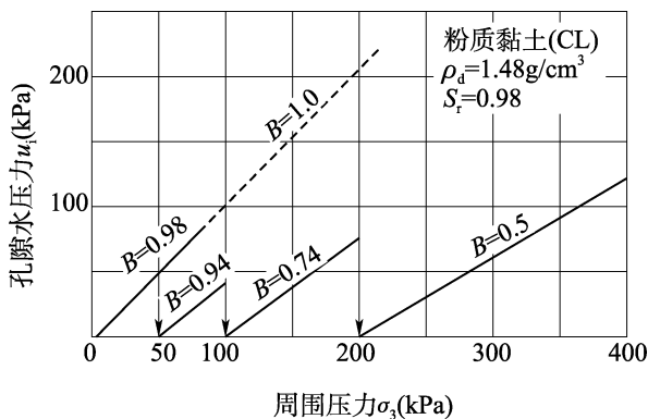
图 4.28.5-2 4 次消散试验中的起始孔隙水压力
