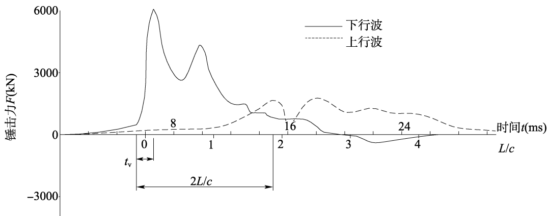
图 6.2.10-2 下行波法确定桩身波速示意图
