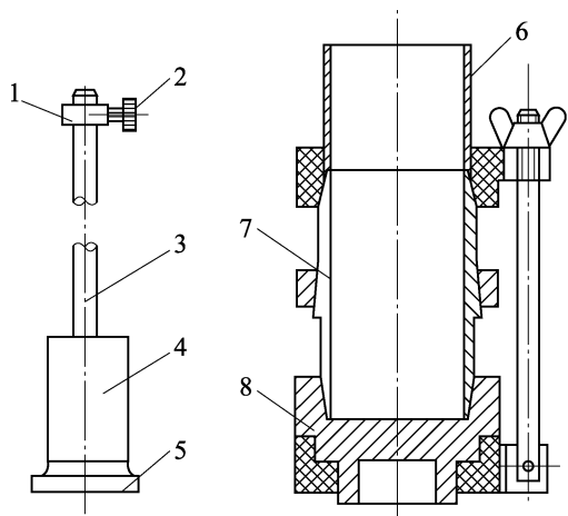
图 4.26.2-2 击样器
