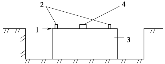
图 7.13.4-2 水平回转振动测试布置图
