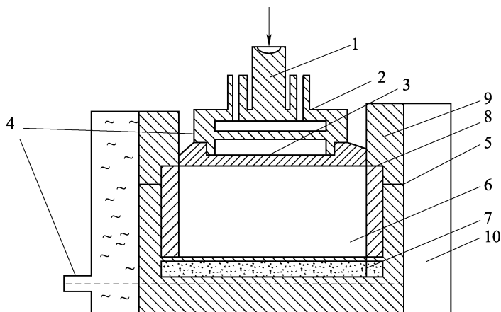
图 4.39.2 融化压缩仪示意图
