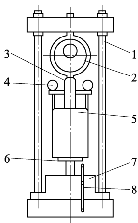
图 4.22.3-3 贯入仪
