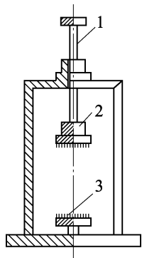
图 4.26.2-4 切土盘 1-转轴;2-上盘;3-下盘
