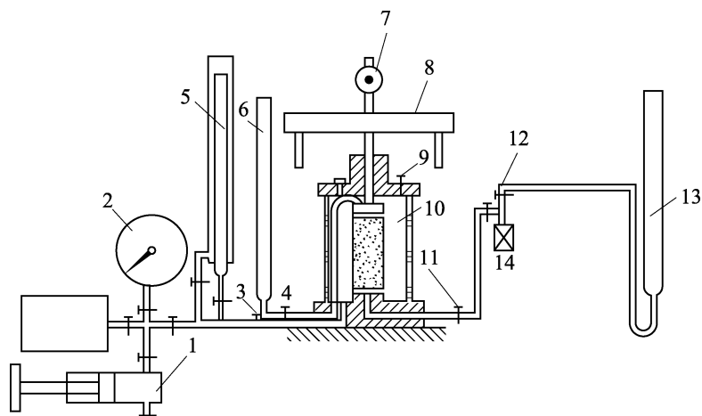
图 4.37.2 应力控制式三轴仪装置
