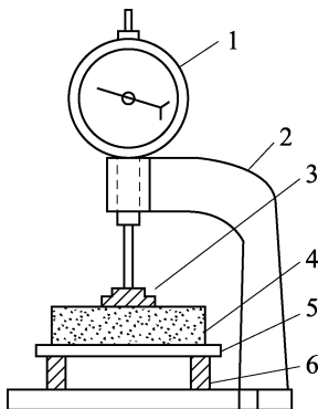
图 4.31.2 收缩仪
