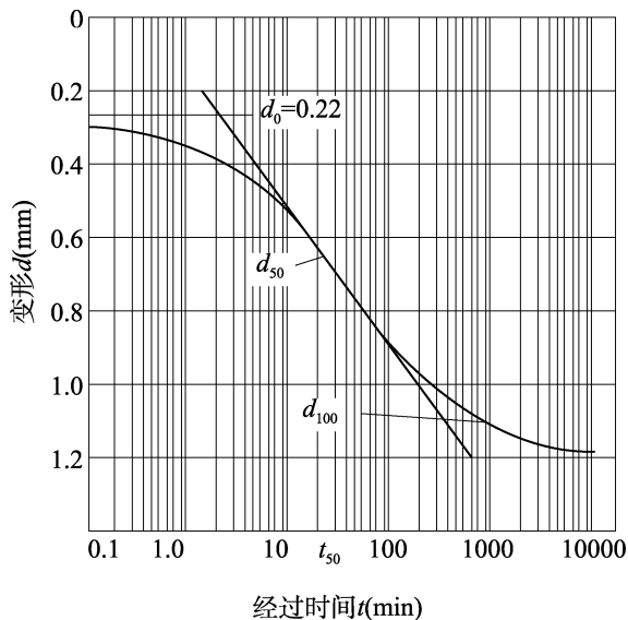
图 4.25.4-4 时间对数法求 t_{50}
