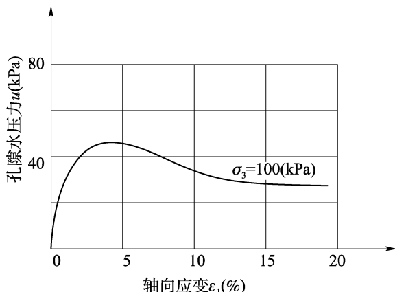
图 4.26.5-4 孔隙水压力与轴向应变关系曲线
