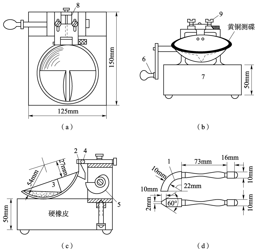
图 4.7.3-1 碟式液限仪
