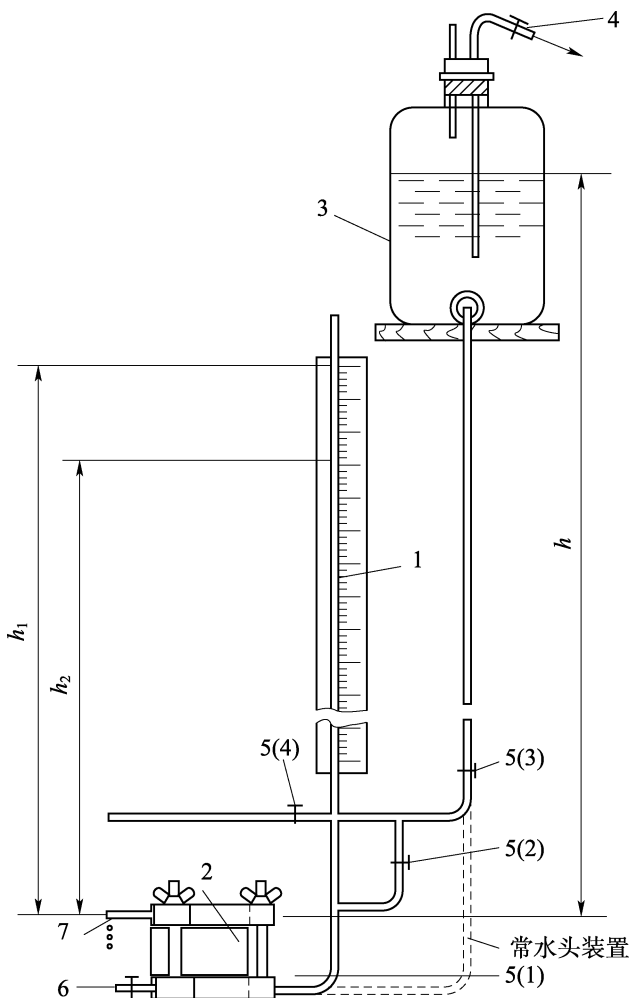
图 4.24.4 变水头渗透装置
