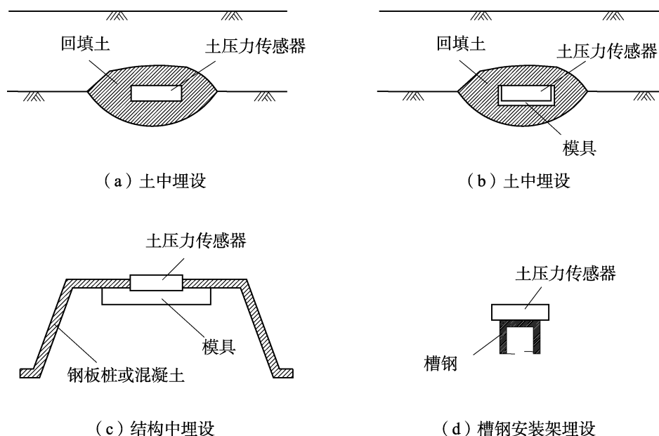
图7-1 几种常见的土压力传感器埋设形式
