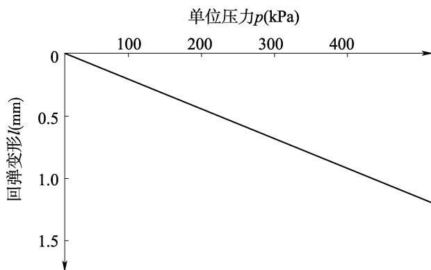
图 4.23.2-3 单位压力与回弹变形 ( p \sim l ) 的关系曲线
