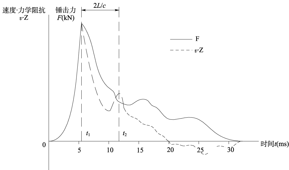
图 6.2.10-1 速度波法确定桩身波速示意图
