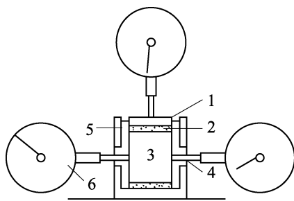
图 4.19.3-1 自由膨胀率试验仪
