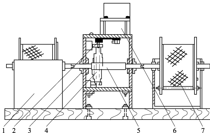
图4.18.2 耐崩解性试验仪
