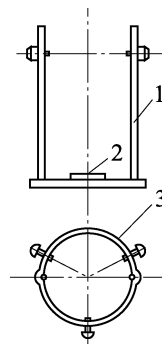
图 4.26.2-6 分样器 1-滑杆;2-底座;3-钢丝架
