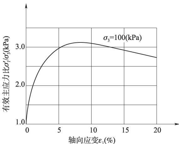
图 4.26.5-3 有效主应力比与轴向应变关系曲线
