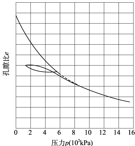
图 4.25.4-1 e \sim p 关系曲线
