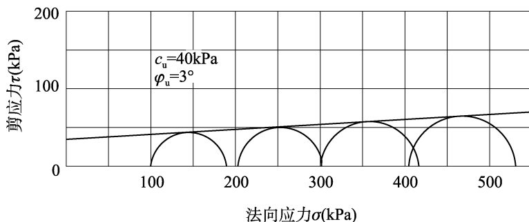
图 4.26.4-2 不固结不排水剪强度包线
