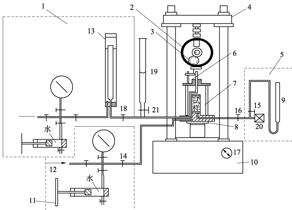
图 4.26.2-1 三轴仪组成示意图
