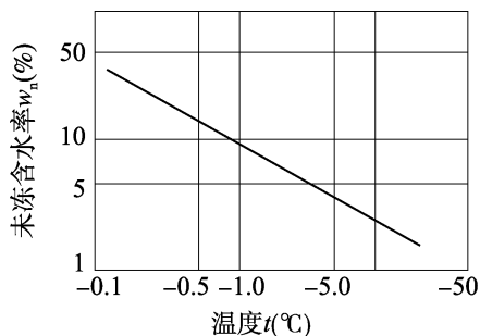
图4.14.5 未冻含水率与温度的关系
