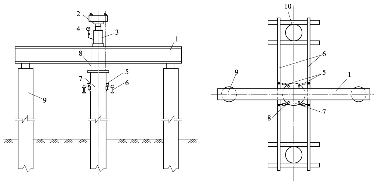
图 6.5.7 锚桩法轴向抗拔静载试验装置
