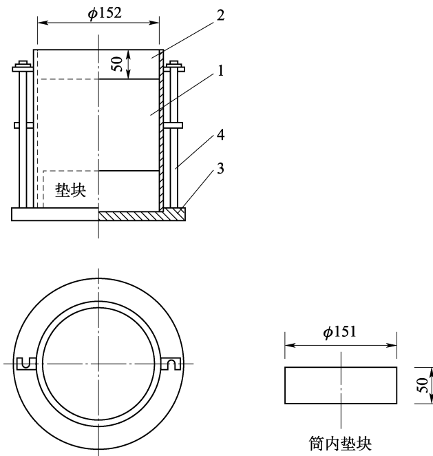
图 4.22.3-1 承载比试筒(单位:mm)
