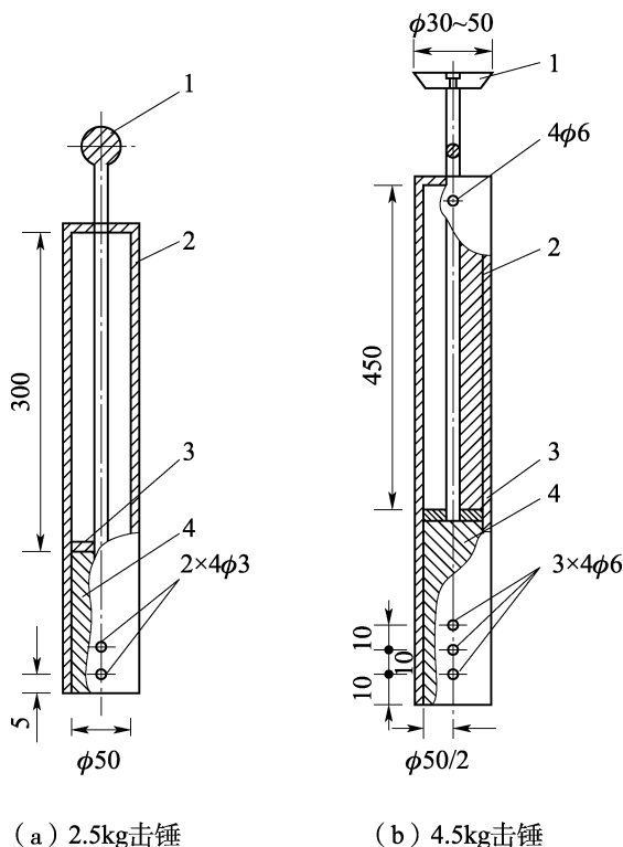
图 4.21.5-2 击锤和导杆 (单位: mm)
