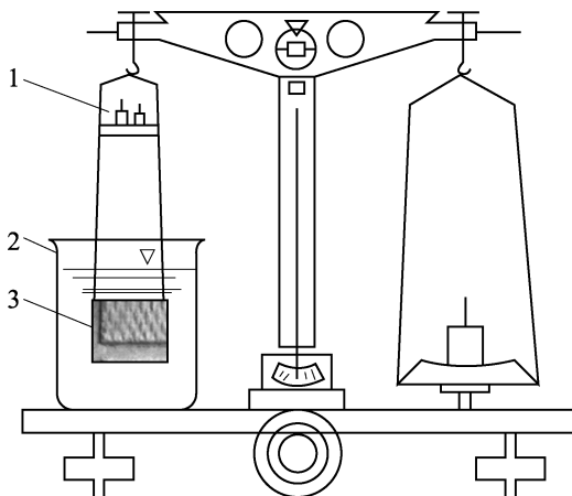
图 4.5.4 浮称法示意图
