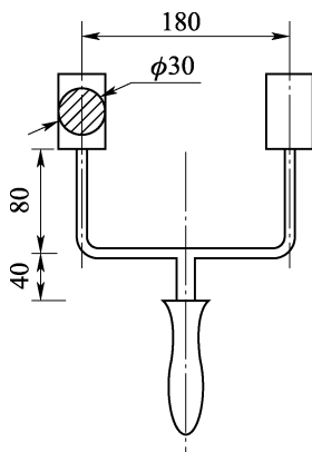
图 4.8.2-2 振动仪(单位:mm)
