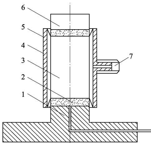
图 4.26.2-7 承膜筒安装示意图
