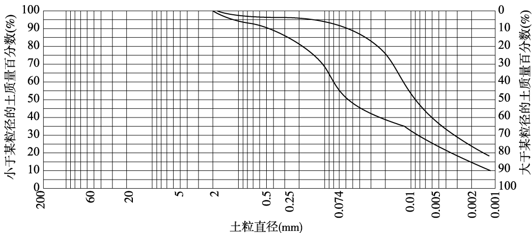
图 4.6.3 粒径分配曲线图
