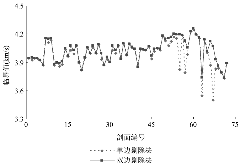
图 6-2 双边法与单边法的临界值
