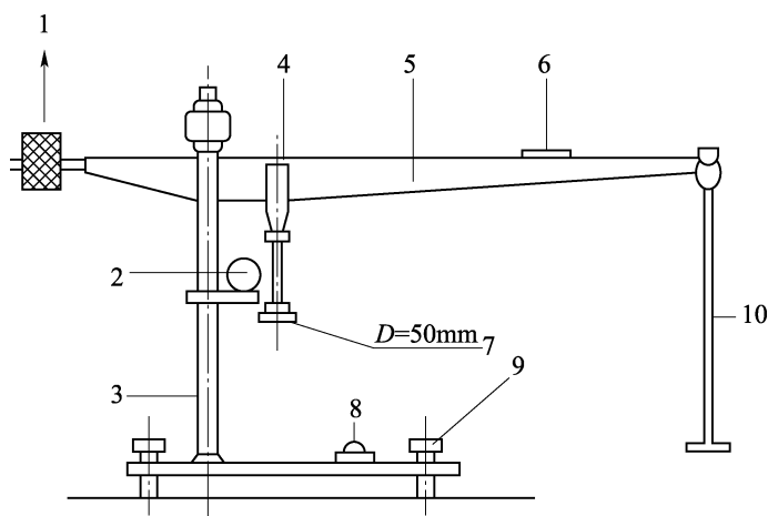
图 4.23.2-1 杠杆压力仪
