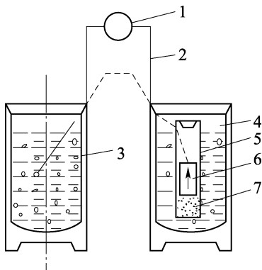
图 4.13.2 冻结温度试验装置示意图
