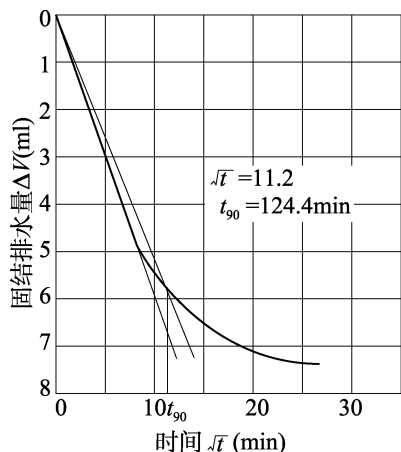
(a) 固结排水量与时间平方根曲线
