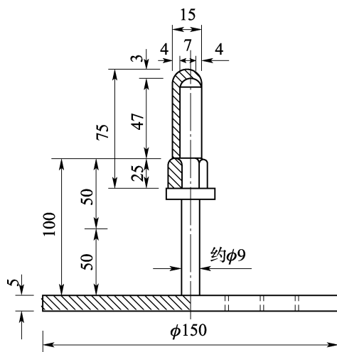
图 4.22.3-4 带调节杆的多孔板(单位:mm)
