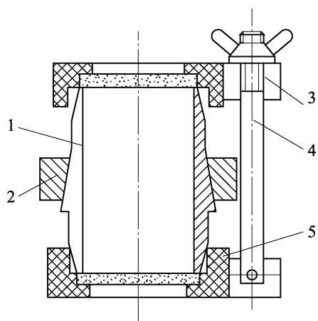
图 4.26.2-3 饱和器
