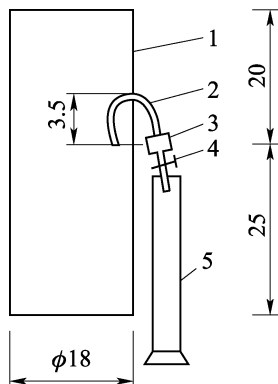
图 4.5.5 虹吸筒(单位:cm)
