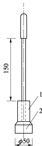
图 4.8.2-3 击锤(单位:mm)
