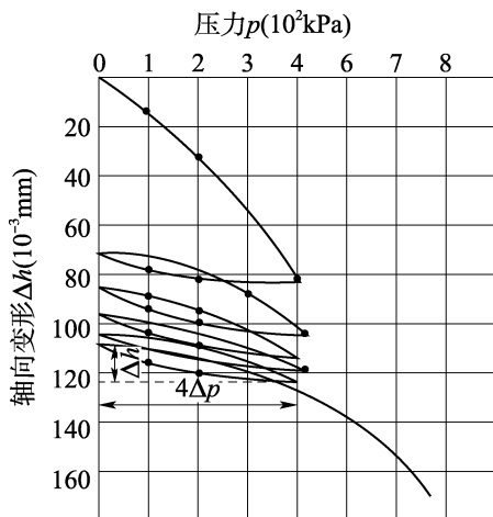
图 4.37.4 加压、卸压与轴向变形关系曲线
