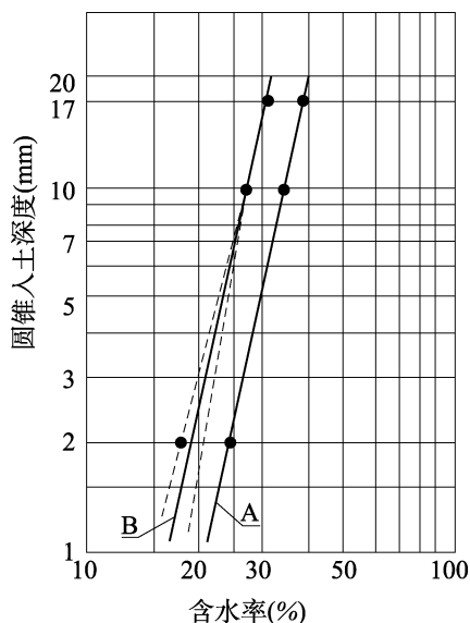
图 4.7.2 h-w 关系图
