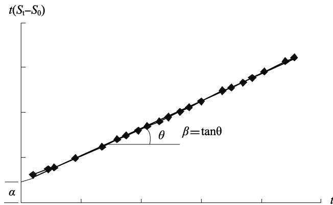
图 7.2.14 图解法求解 \alpha, \beta 值
