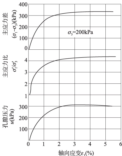
图 4.26.7-2 固结不排水剪应力与应变曲线
