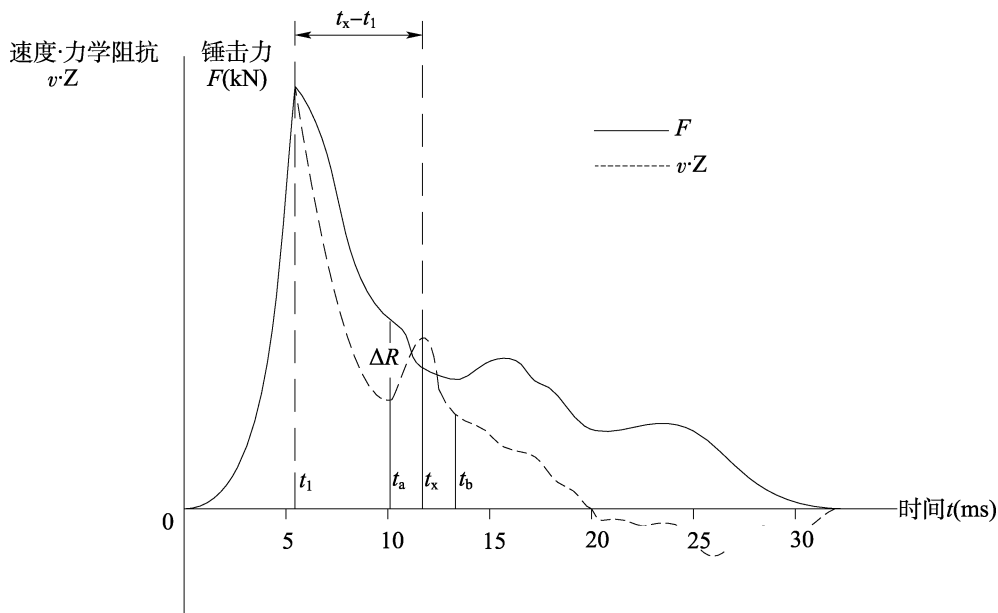
图 6.2.14 桩身完整性系数计算示意图
