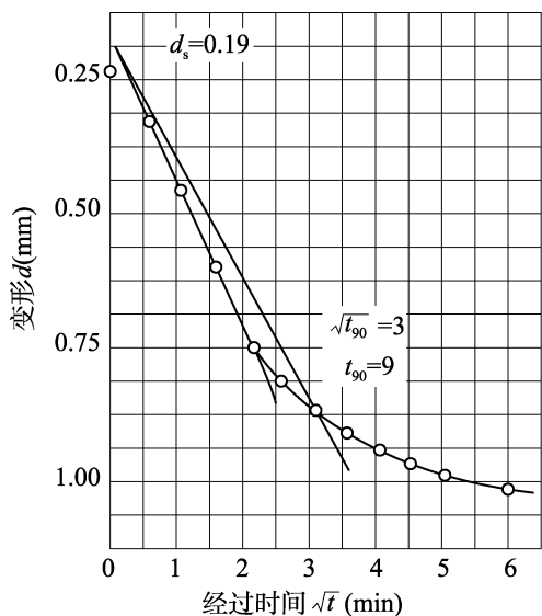
图 4.25.4-3 时间平方根法求 t_{90}
