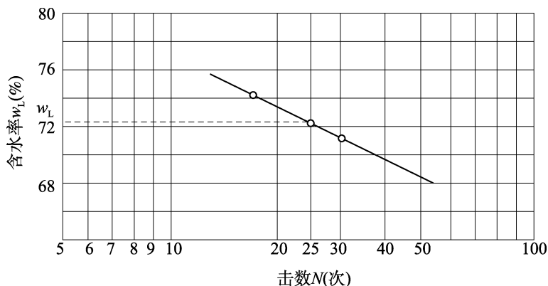
图 4.7.3-2 含水率与击数关系曲线
