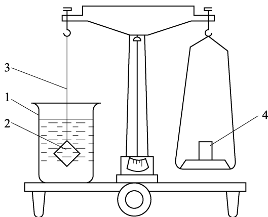
图 4.12.2 浮称法示意图
