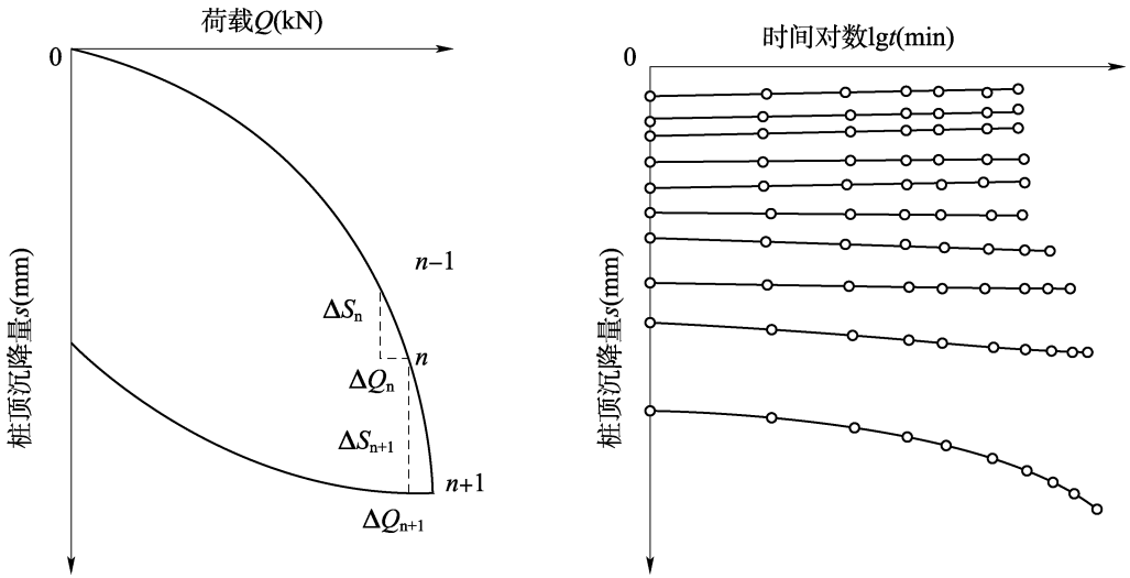
(a) 有陡降段的 Q\sim s 曲线
