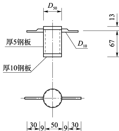
图 4.23.2-2 承载板(单位:mm)
