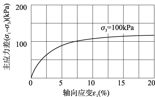
图 4.26.4-1 主应力差与轴向应变关系曲线
