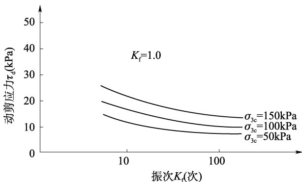
图 4.27.4-1 动剪应力与振次关系曲线
