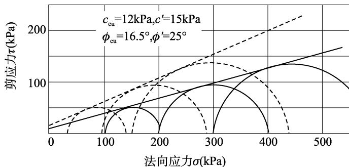
图 4.26.5-6 固结不排水剪强度包线
