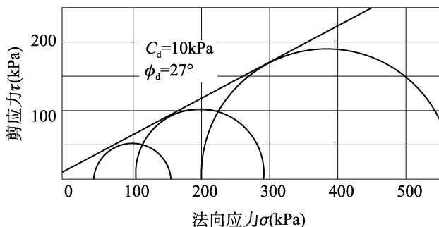
图 4.26.6 固结排水剪强度包线
