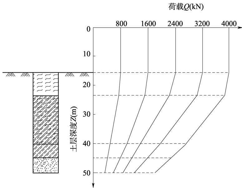
图 6.4.18 桩身轴向力分布
