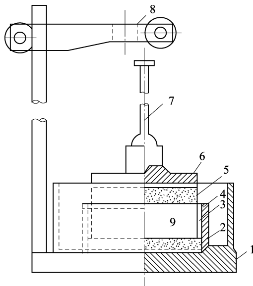
图 4.25.2 固结容器示意图
