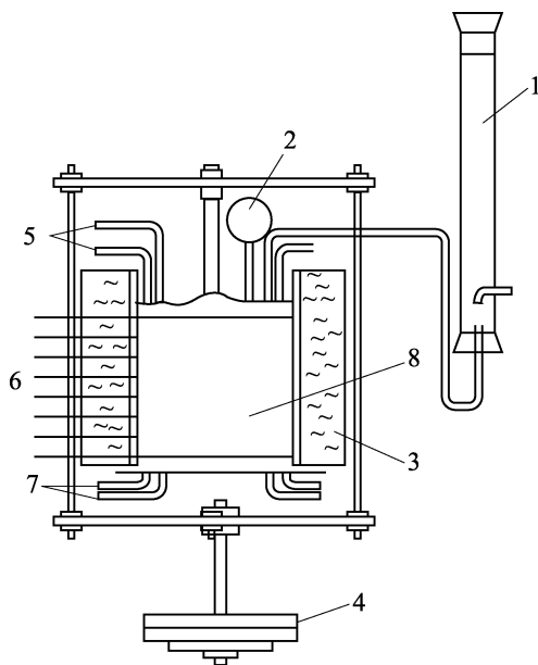
图 4.38.2 试样盒结构示意图
