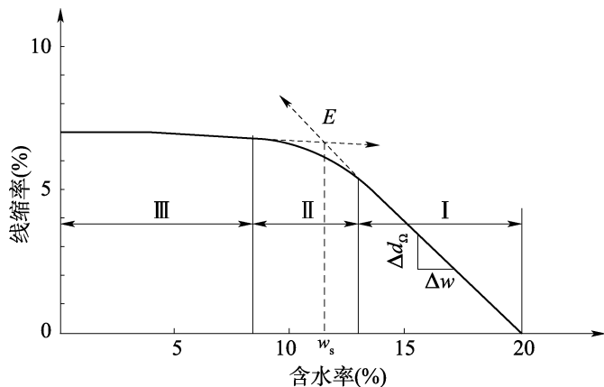
图 4.31.7 线缩率与含水率关系曲线
