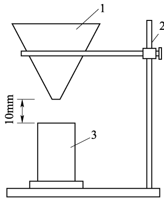
图 4.32.2-2 量样装置
