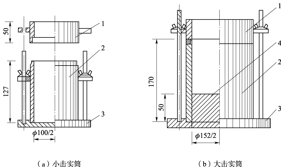
图 4.21.5-1 击实筒(单位:mm)
