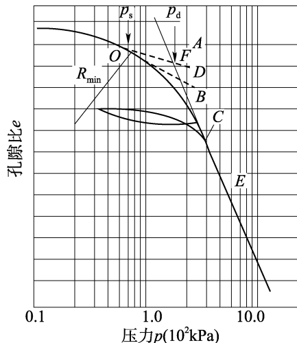
图 4.25.4-2 e \sim \lg p 曲线和求 p_c 示意图
