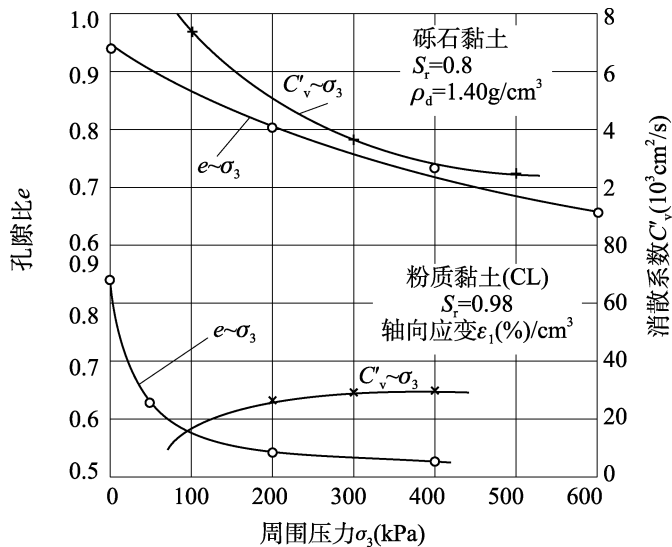
图 4.28.5-4 孔隙比、消散系数与压力曲线
