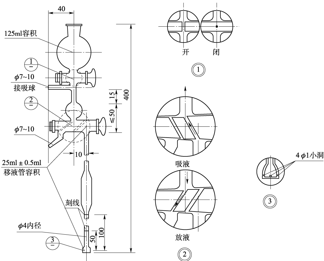
图 4.6.4 移液管(单位:mm)
