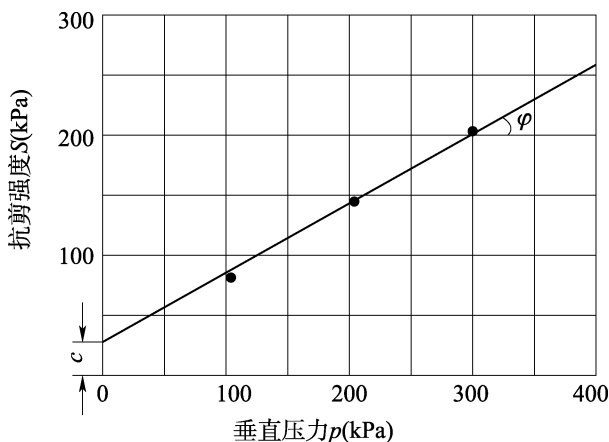
图 4.30.7 抗剪强度与垂直压力关系曲线
