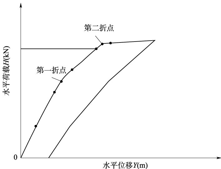
图 6.6.18 水平荷载-力作用点位移关系( H \sim Y )曲线
