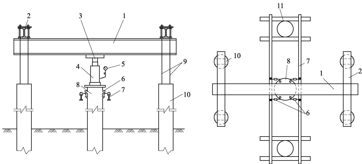
图 6.4.13 锚桩法轴向抗压静载试验装置
