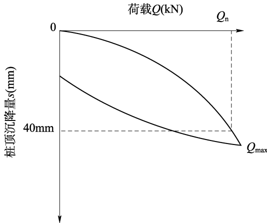
(c) 无明显陡降段的 Q\sim s 曲线
