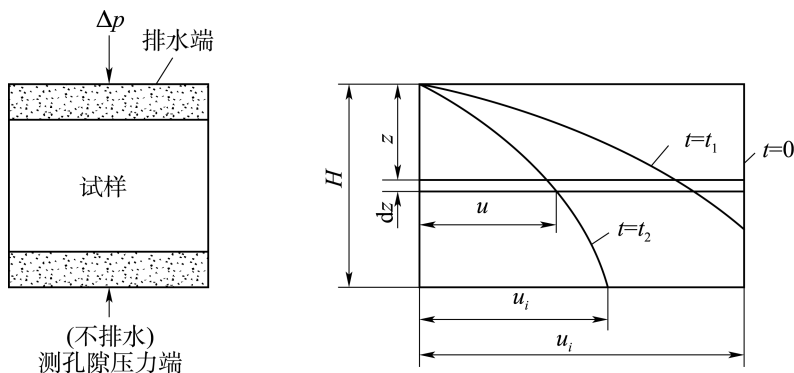
图 4-2 试样布置及孔隙水压力分布线图
