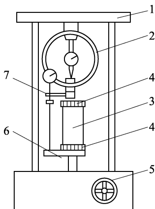
图 4.29.2 应变控制式无侧限压缩仪
