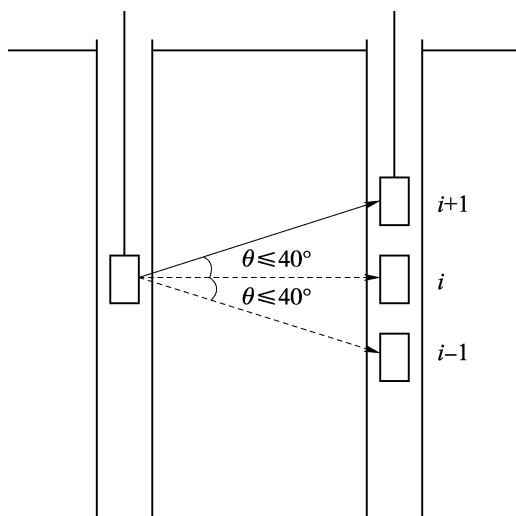
图 6.8.9 扇形扫测示意图
