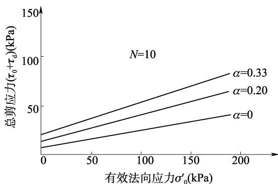
图 4.27.4-2 总剪应力与有效法向应力关系曲线
