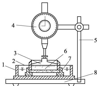
图 4.19.3-2 侧向约束膨胀率试验仪
