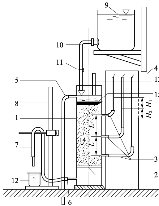
图 4.24.3-1 常水头渗透仪装置
