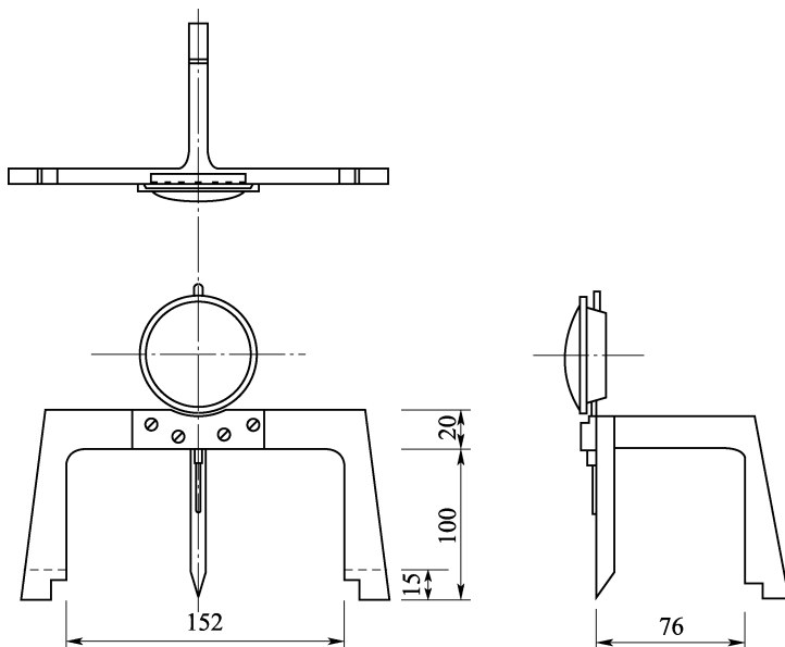
图 4.22.3-2 膨胀量测定装置(单位:mm)(仅供参考)——QQ群: 868029499
