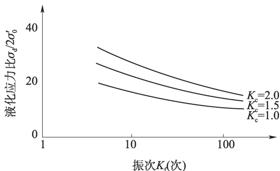
图 4.27.4-3 液化应力比与振次关系曲线
