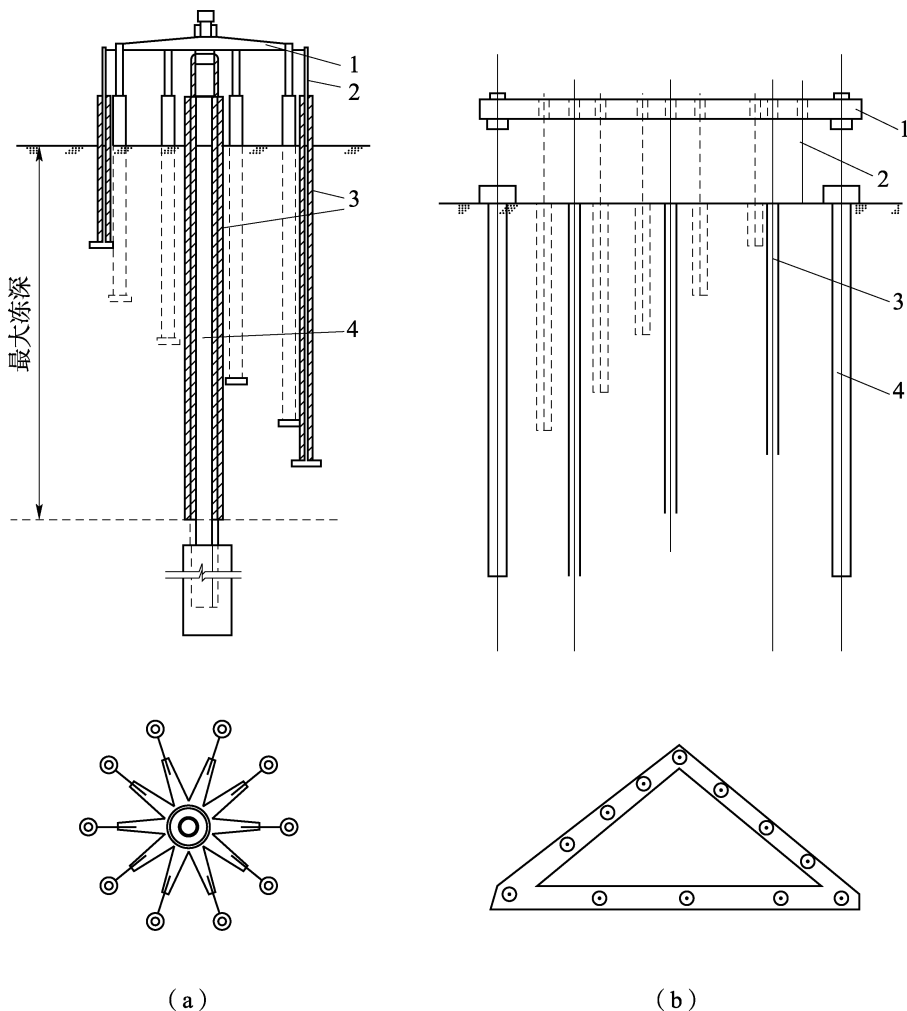
图 5.6.2 分层冻胀仪示意图
