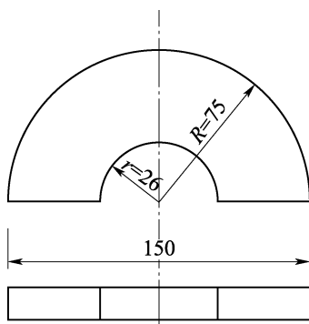
图 4.22.3-5 荷载块(单位:mm)
