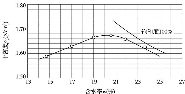
图 4.21.8 含水率与干密度的关系曲线
