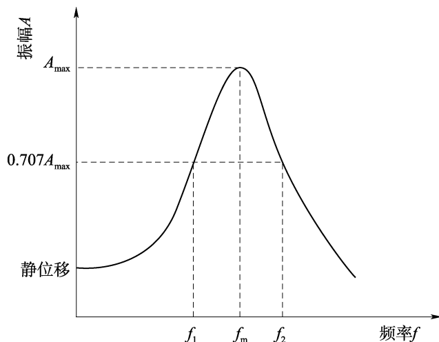
图 4.36.7 稳态强迫振动振幅与频率关系曲线
