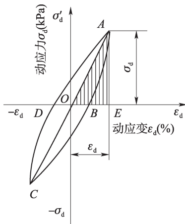
图 4.27.4-5 应力应变滞回圈
