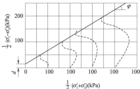
图 4.26.5-5 应力路径曲线 (正常固结黏土)
