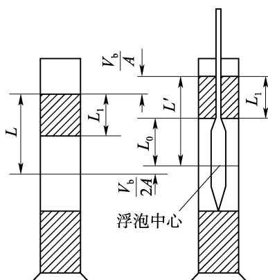
图 4-1 土粒有效沉降距离校正
