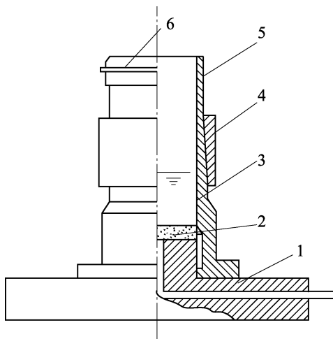
图 4.26.2-8 制备砂样圆模
