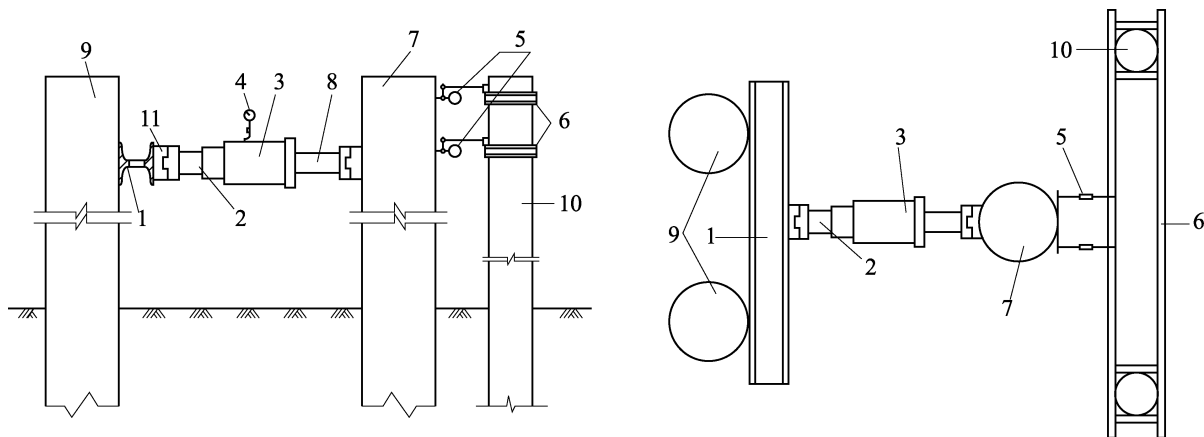
图 6.6.15 水平静载试验装置图
