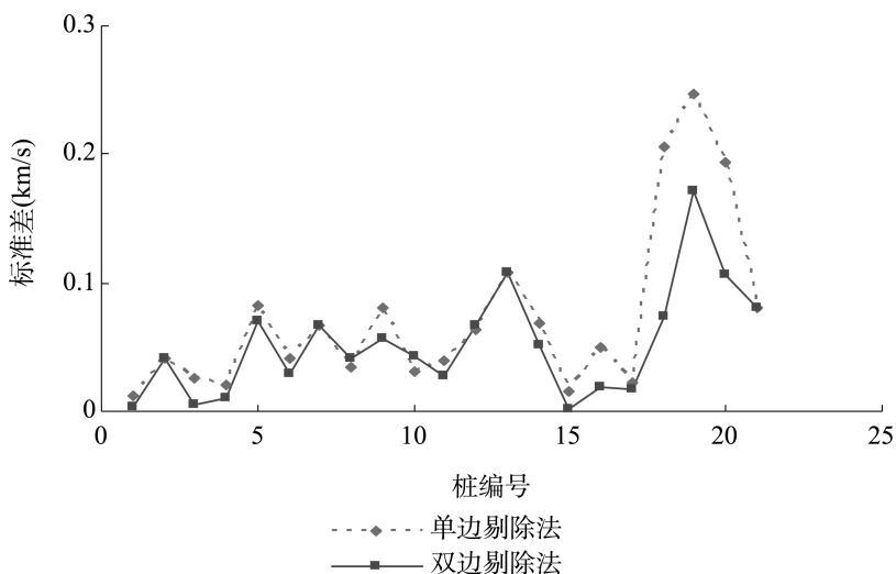
图 6-3 双边法与单边法的标准差
