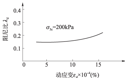
图 4.27.4-6 阻尼比与动应变关系曲线
