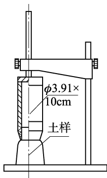
图 4.26.2-5 切土器和切土架
