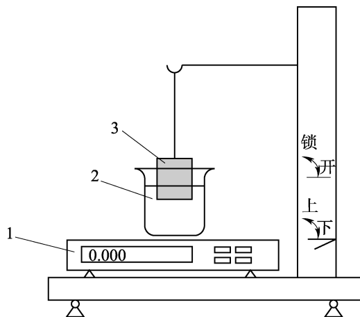
图 4.5.3 浮力法示意图
