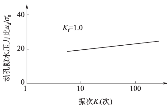
图 4.27.4-4 动孔隙水压力比与振次关系曲线
