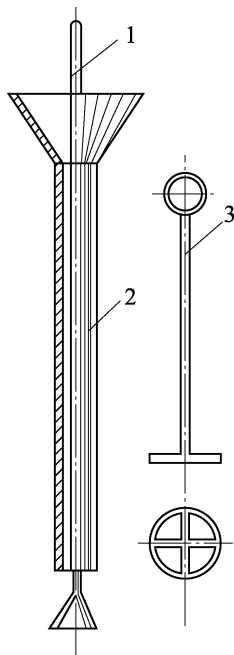
图 4.8.2-1 长颈漏斗
