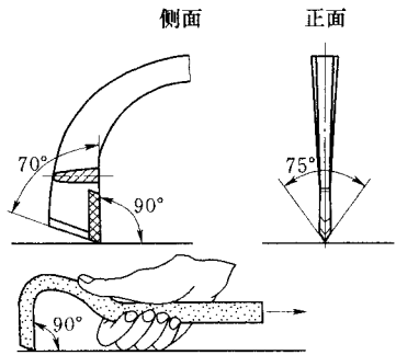
图 G.2.2 切割工具
