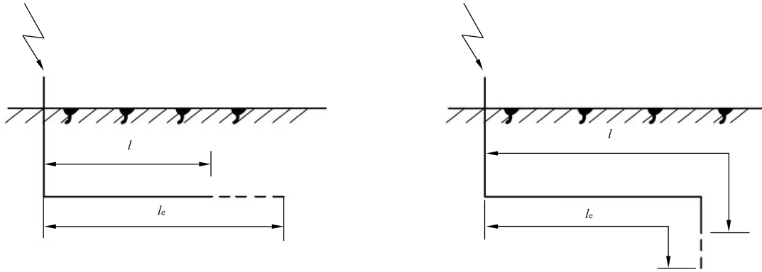
a) 单根水平接地体
