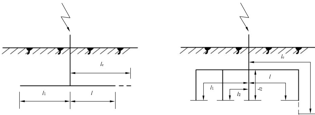
c) 多根水平接地体, l_1 \leq l
