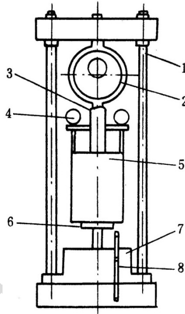
图 T0134-2 荷载装置示意图
