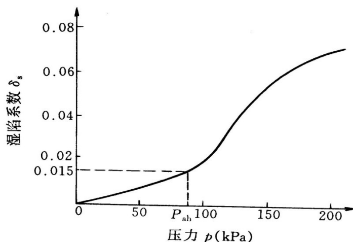
图 T0175-1 湿陷系数与压力关系曲线
