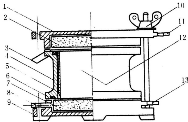
图 T 0130-1 渗透容器
