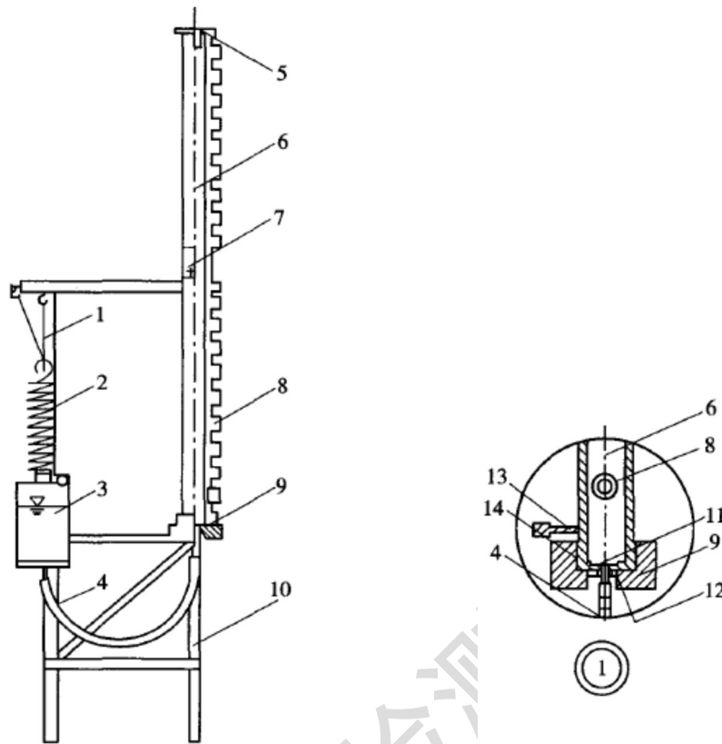
图 T 0128-1 毛细管试验仪
