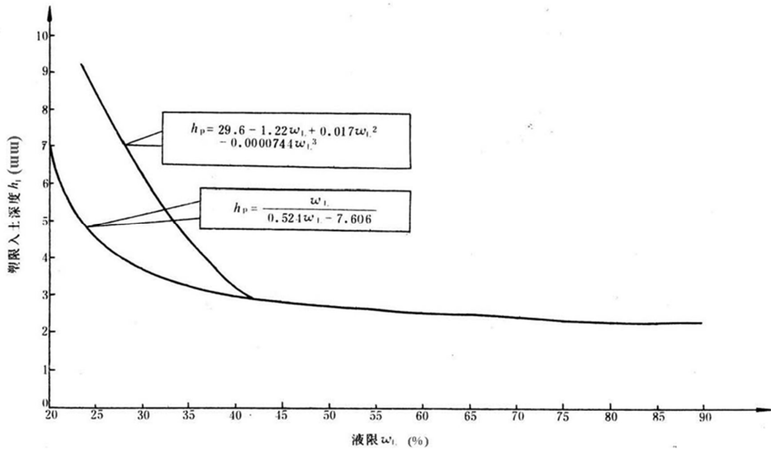
图 T0118-3 h_p - w_L 关系曲线
