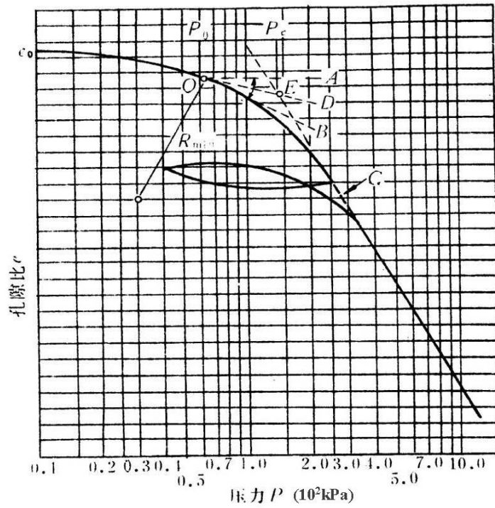
图 T0137-5 e - \lg P 曲线先期固结压力
