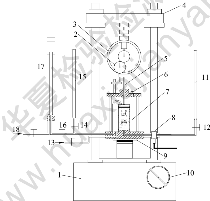
图 T0144-1 应变控制式三轴压缩仪示意图
