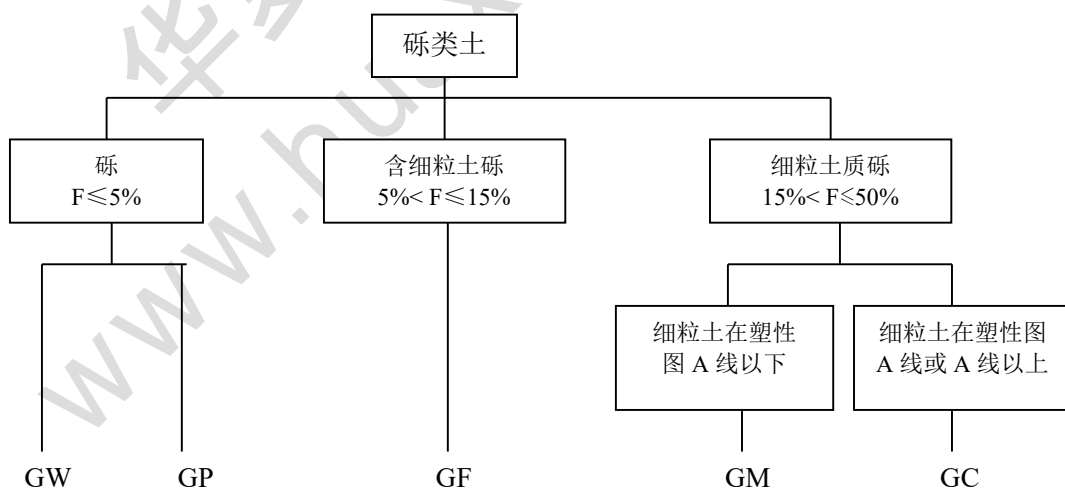
图 3.3.2 砾类土分类体系
