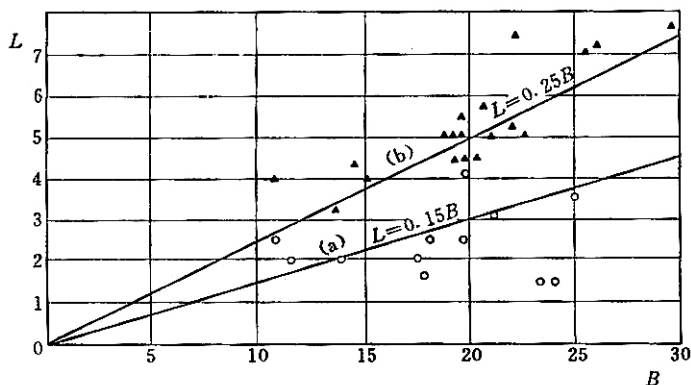
图 1 部分工程锚杆长度与开挖跨度关系
