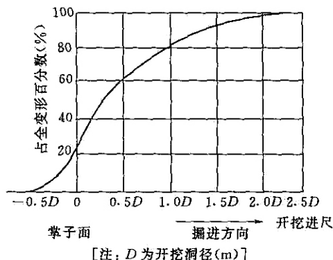
图 4 开挖过程典型收敛曲线
