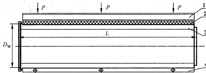
a) PCCPL 管外压荷载试验示意图
