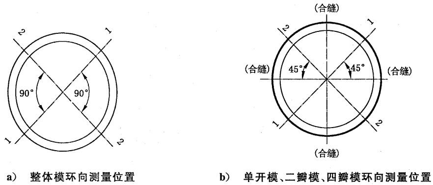
图 3 直径环向测量位置示意图
