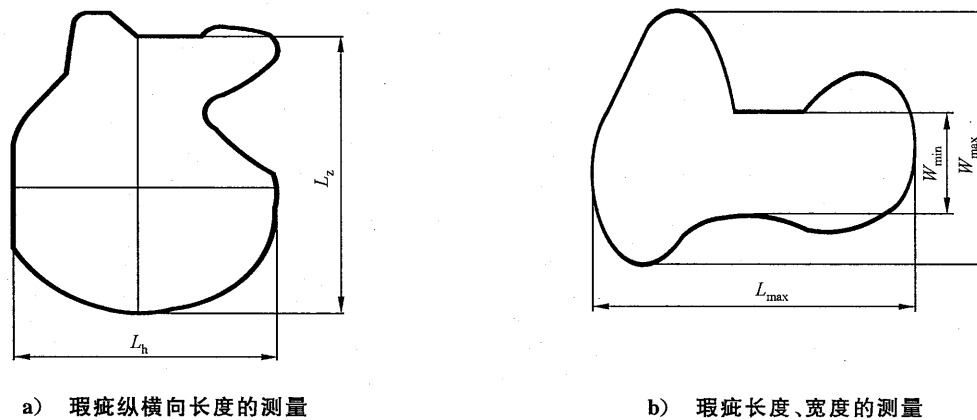
图 1 瑕疵尺寸测量示意图
