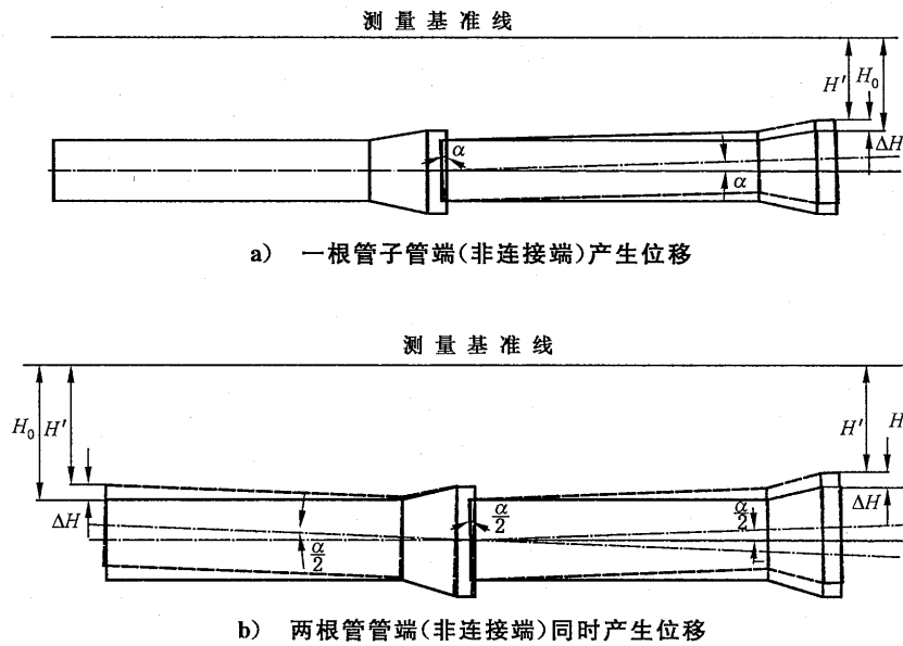
图 12 管子接头相对转角密封性能试验示意图
