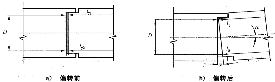
图 13 管子转角接头密封性能试验示意图
