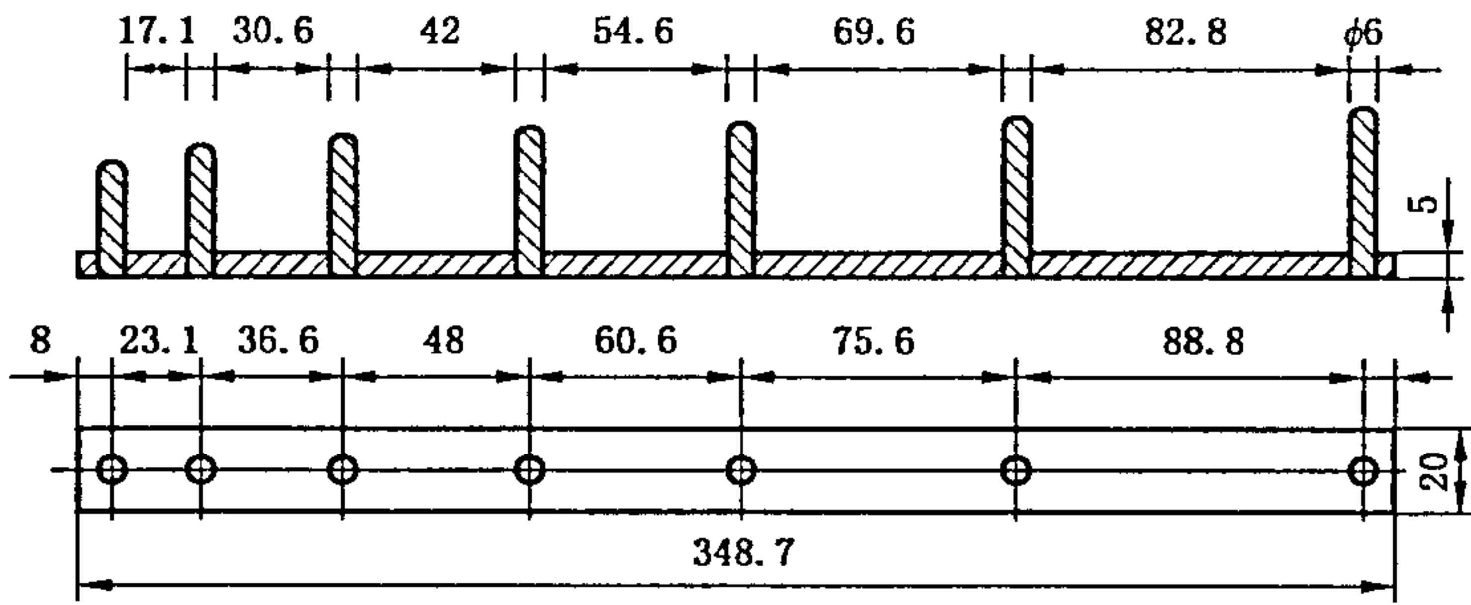
图 1 针状规准仪
