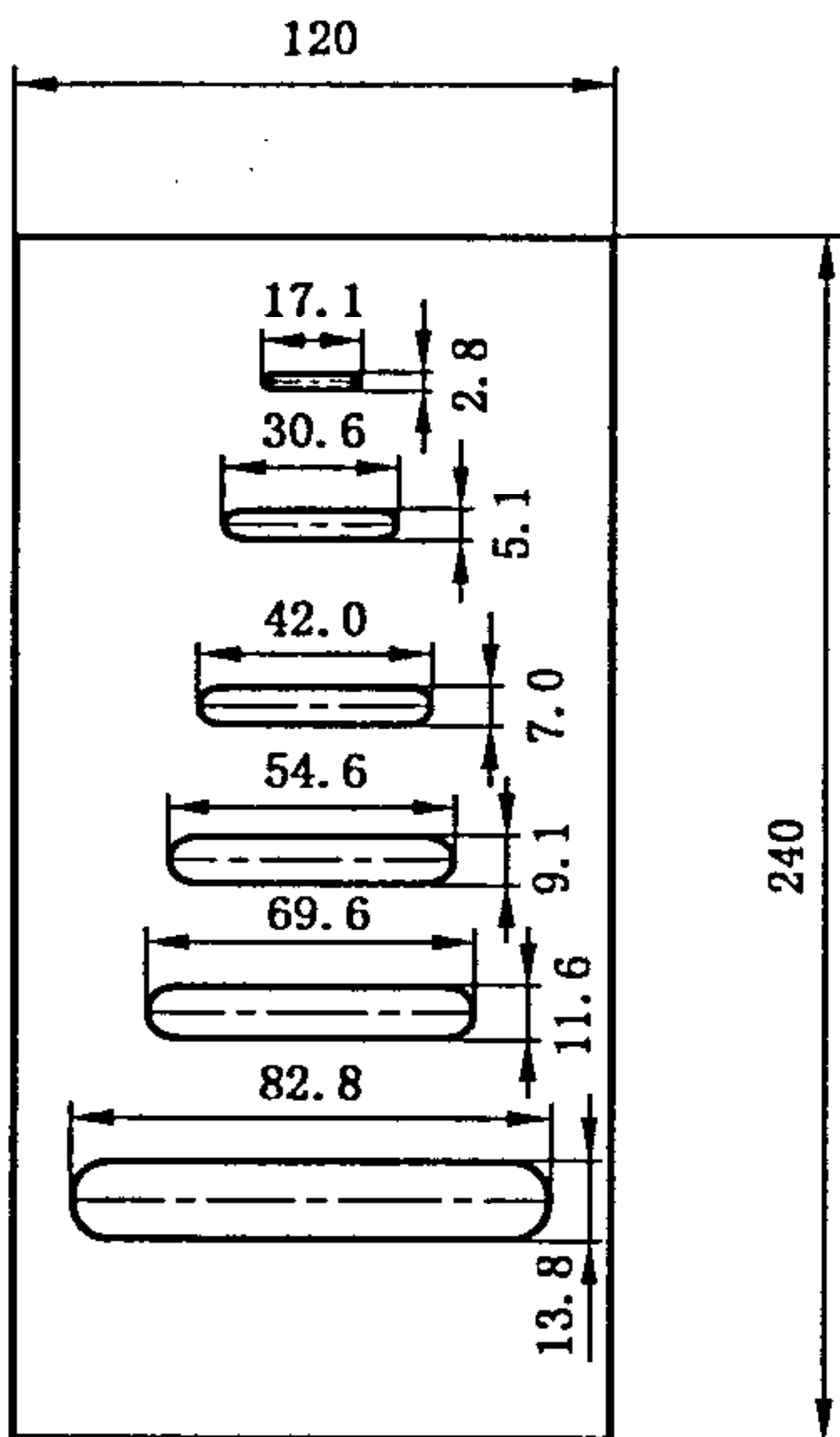
图 2 片状规准仪
