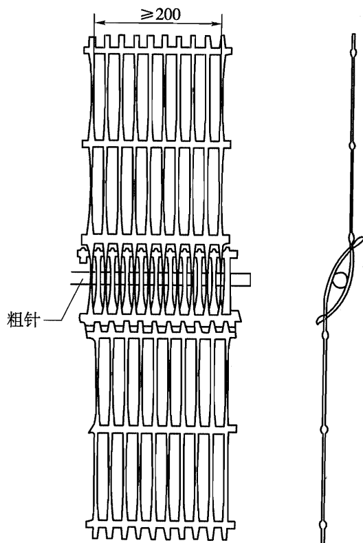
图 T 1122-2 土工格栅试样图(尺寸单位:mm)
