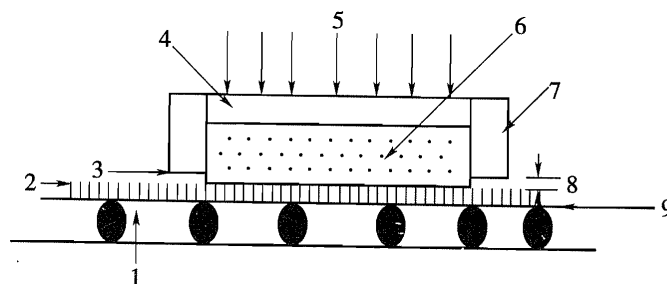
图 T 1129-1 接触面积不变直剪仪示意图
