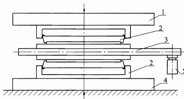
图 E.1 成品支座转动试验装置
