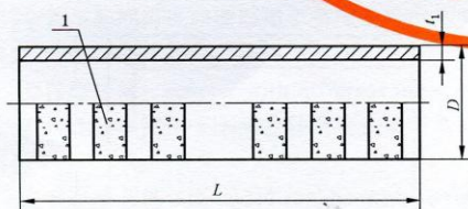
a) 挤压标准型套筒
