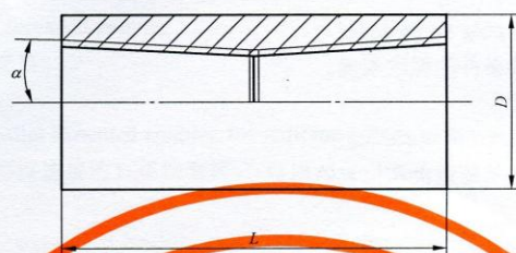
a) 锥螺纹标准型套筒
