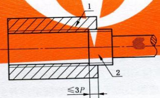
图 4 直螺纹套筒螺纹中径通端检验示意图
