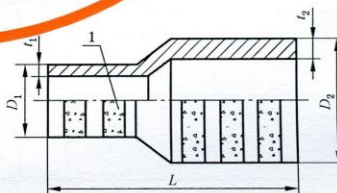
b) 挤压异径型套筒
