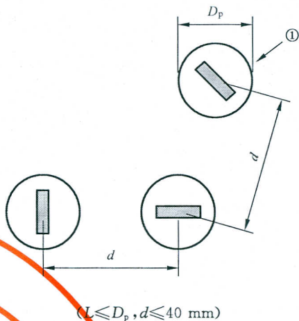
图 7 密集形的不连续
